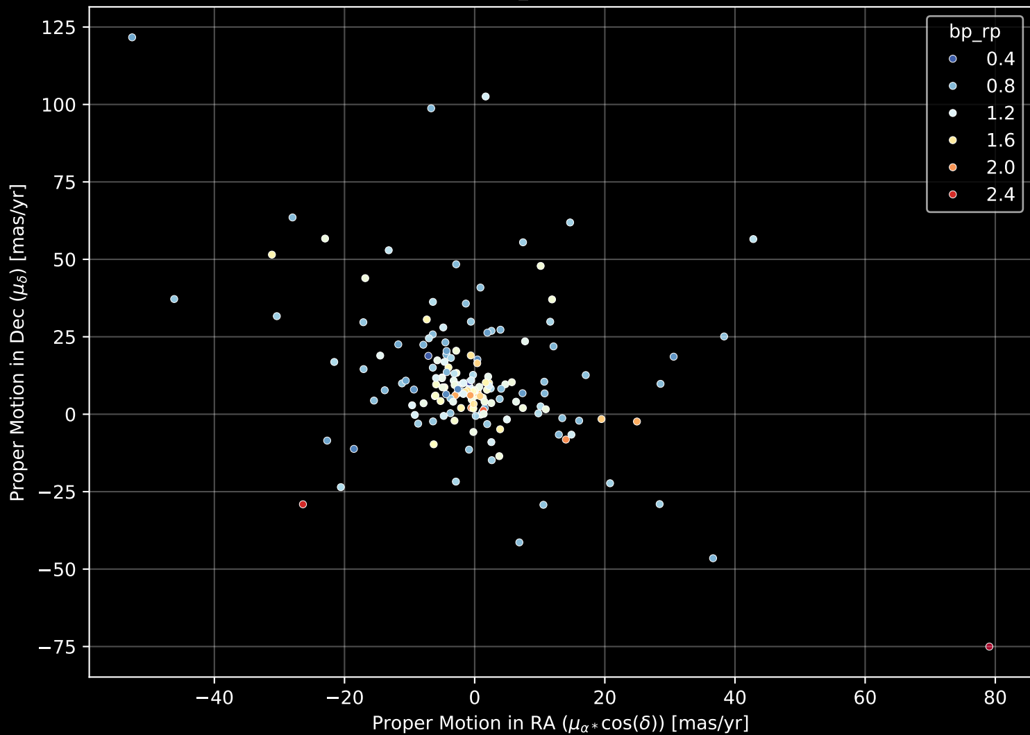
APOGEE DR17 Field: [281-24-O_TESS] Proper Motion Diagram (n= 167)
