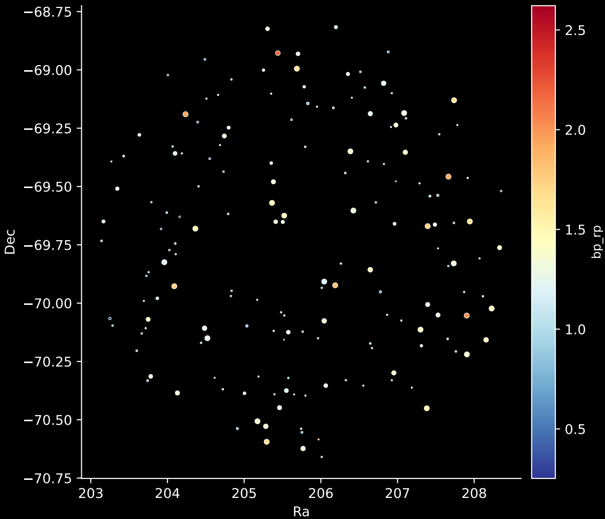
APOGEE DR17 Field: [281-24-O_TESS] Stars: 167
