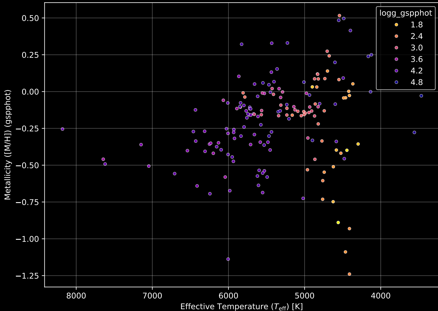
APOGEE DR17 Field: [281-24-O_TESS] Stellar Population Parameters (n= 167)
